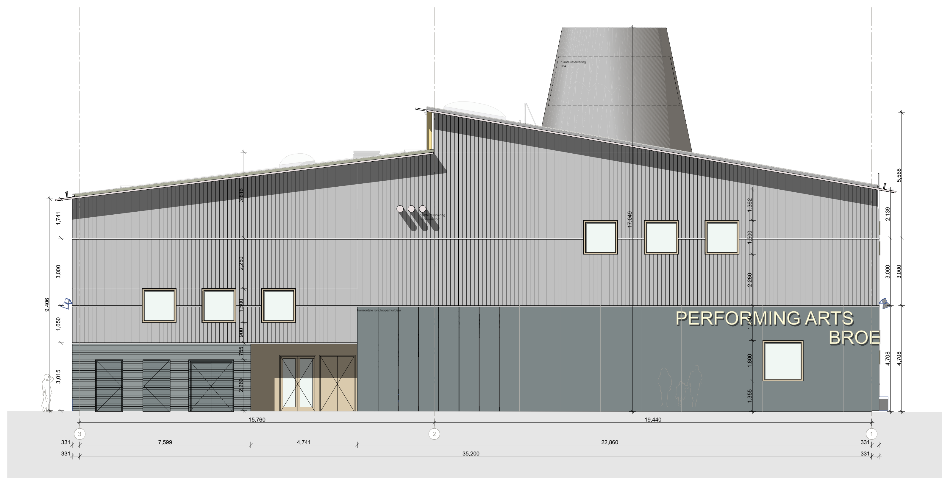
Noordgevel
