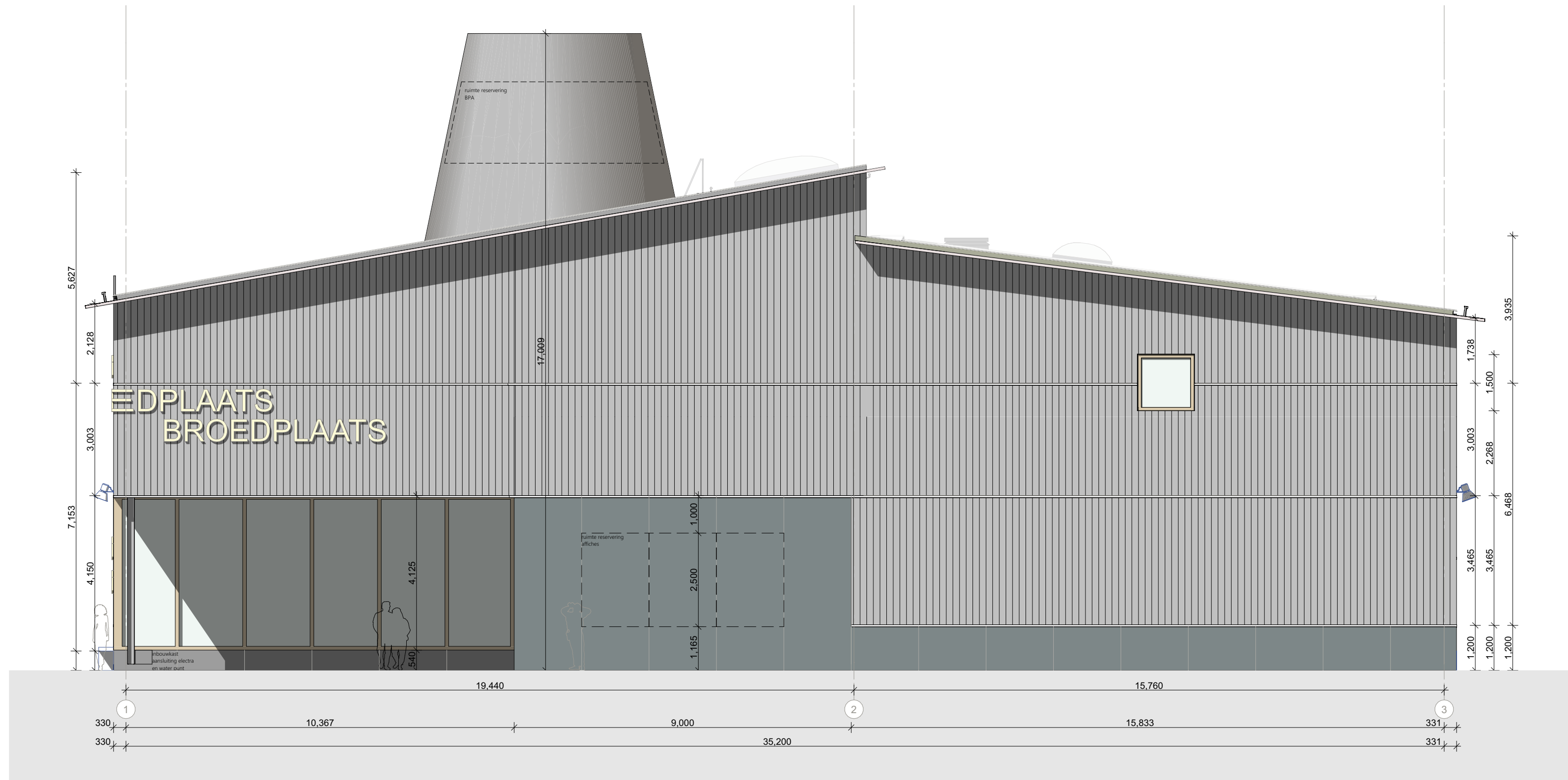
Zuidgevel
